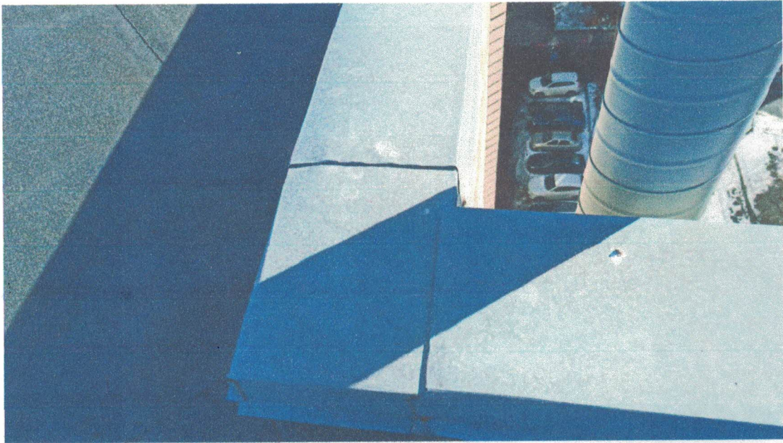
Фото 18. Отсутствует гидроизоляция стыков покрытия парапетов.
